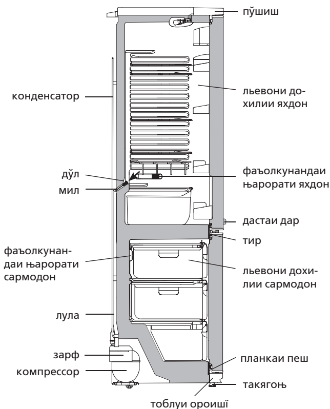
Расми 7 — Наќшаи партоби оби яхшудаи яхдон
